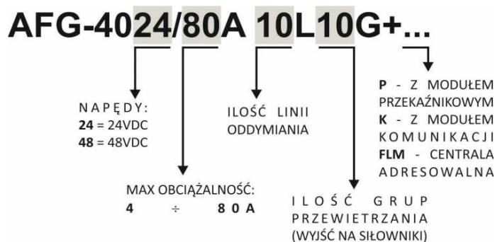
Rysunek 2. Oznaczenie typu, tabliczka znamionowa dla wersji AFG-4024/4048
