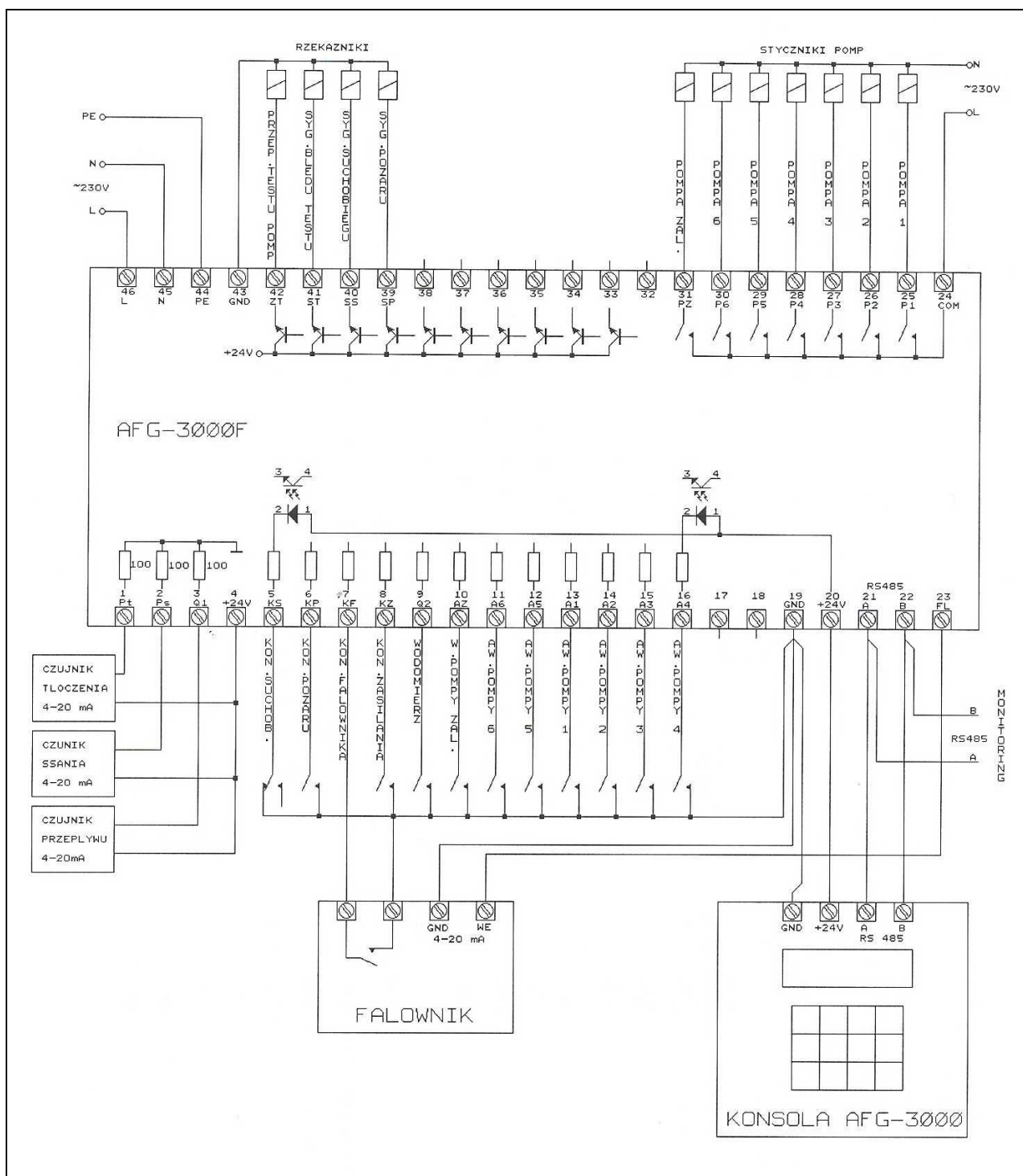
Rysunek 2. Schemat połączeń sterownika AFG-3000F
